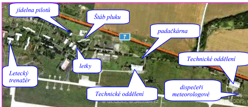
Rozmístění důležitých pracovišť 11.sl.p
